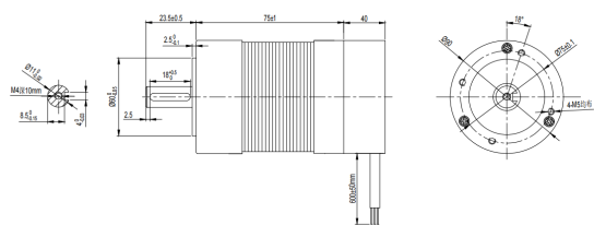
机械尺寸图 DIMENSIONS • unit = mm
